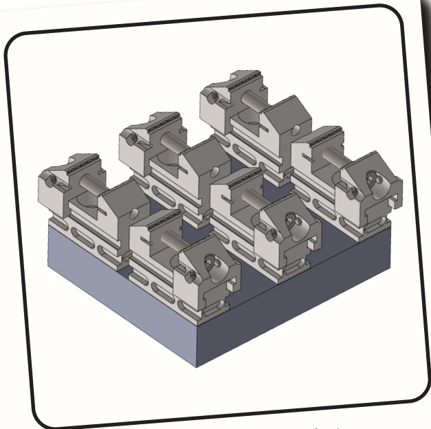
6 x KTS 60 auf einer Palette 6 x KTS 60 on a pallet
